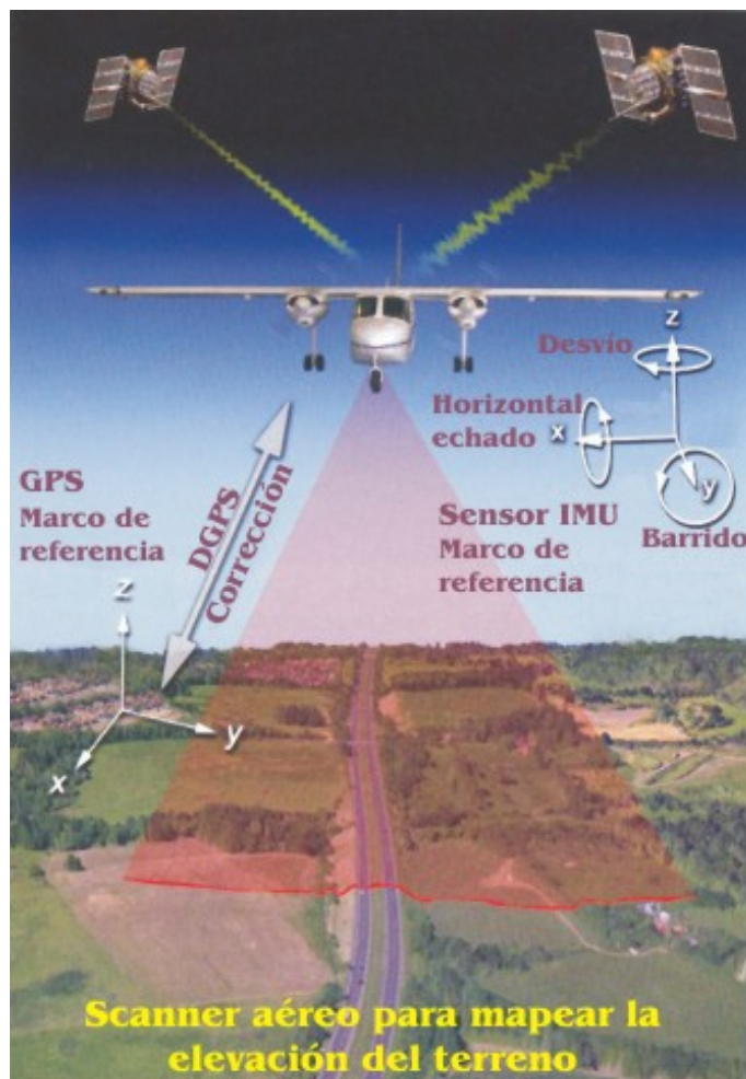
Figura 2.24 Descripción del sistema Lidar
