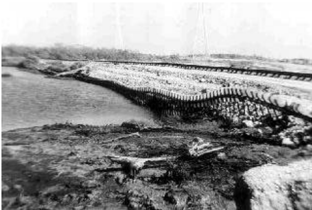
Fig. 20. Daños a la infraestructura por tsunami. Lázaro Cárdenas, México, 1985.
