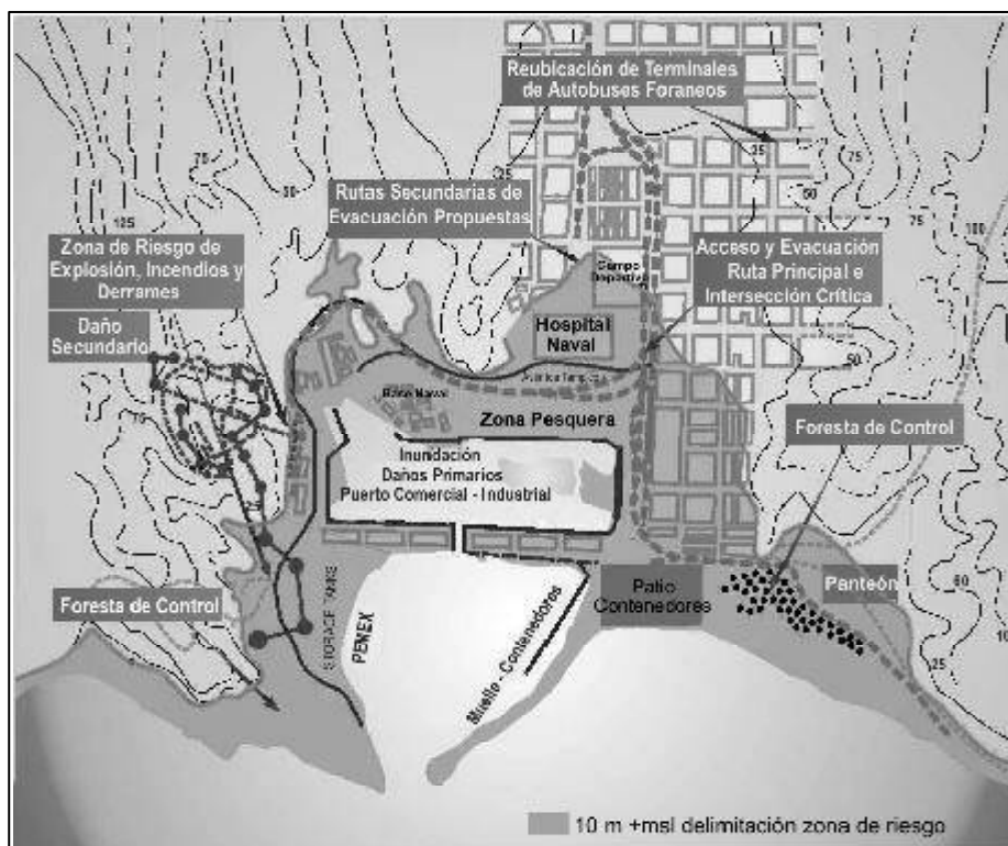
Fig. 37. Salina Cruz, Oax. Análisis de vulnerabilidad según usos del suelo, y recomendaciones para reducción del impacto por tsunamis, en la franja costera delimitada por la cota de 10 metros sobre nivel medio del mar. Fuente: Diagnóstico de Peligros e Identificación de Riesgos de Desastres en México. CENAPRED. México, D.F. 2001.
