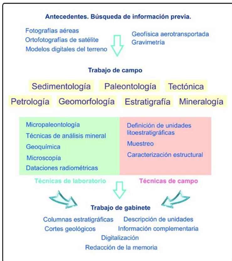
Figura 1. Esquema conceptual simplificado de los pasos y técnicas básicas en la cartografía geológica.
