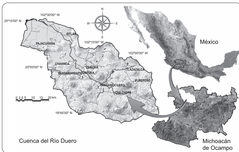
Fig. 1. Ubicación geográfica de la cuenca del río Duero
