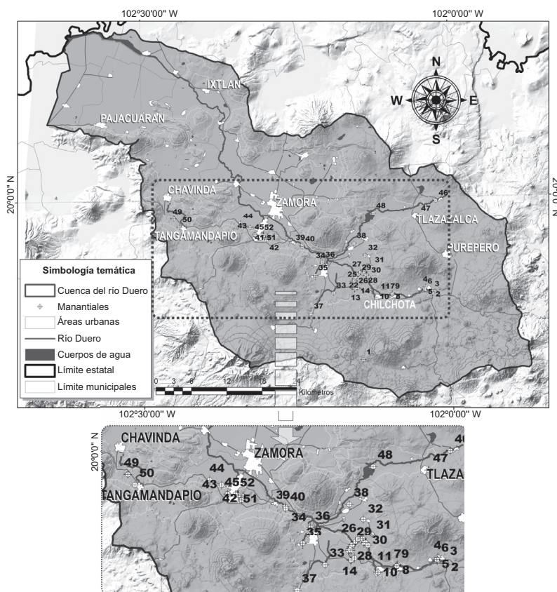
Fig. 4. Localización de los 52 manantiales dentro de la cuenca del río Duero
