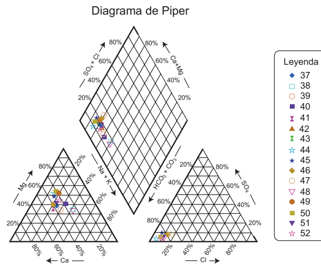
Fig. 5. Clasificación de Piper obtenidos para cada manantial
