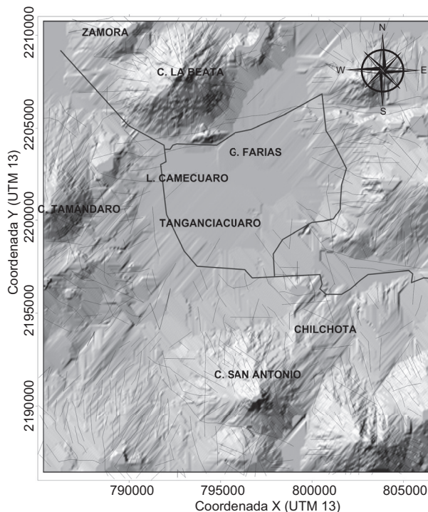
Fig. 2. Esquema representativo del ámbito local estructural de la cuenca del río Duero, Valle de Guadalupe
