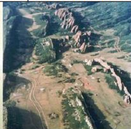
Riscos en capas verticales.
