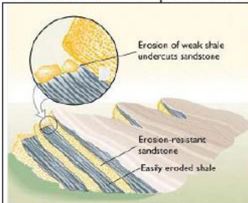
Cuestas en capas inclinadas.
