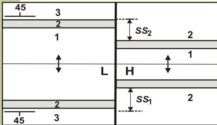
Anticlinal simétrico
