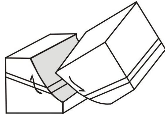
(f) rotacional
