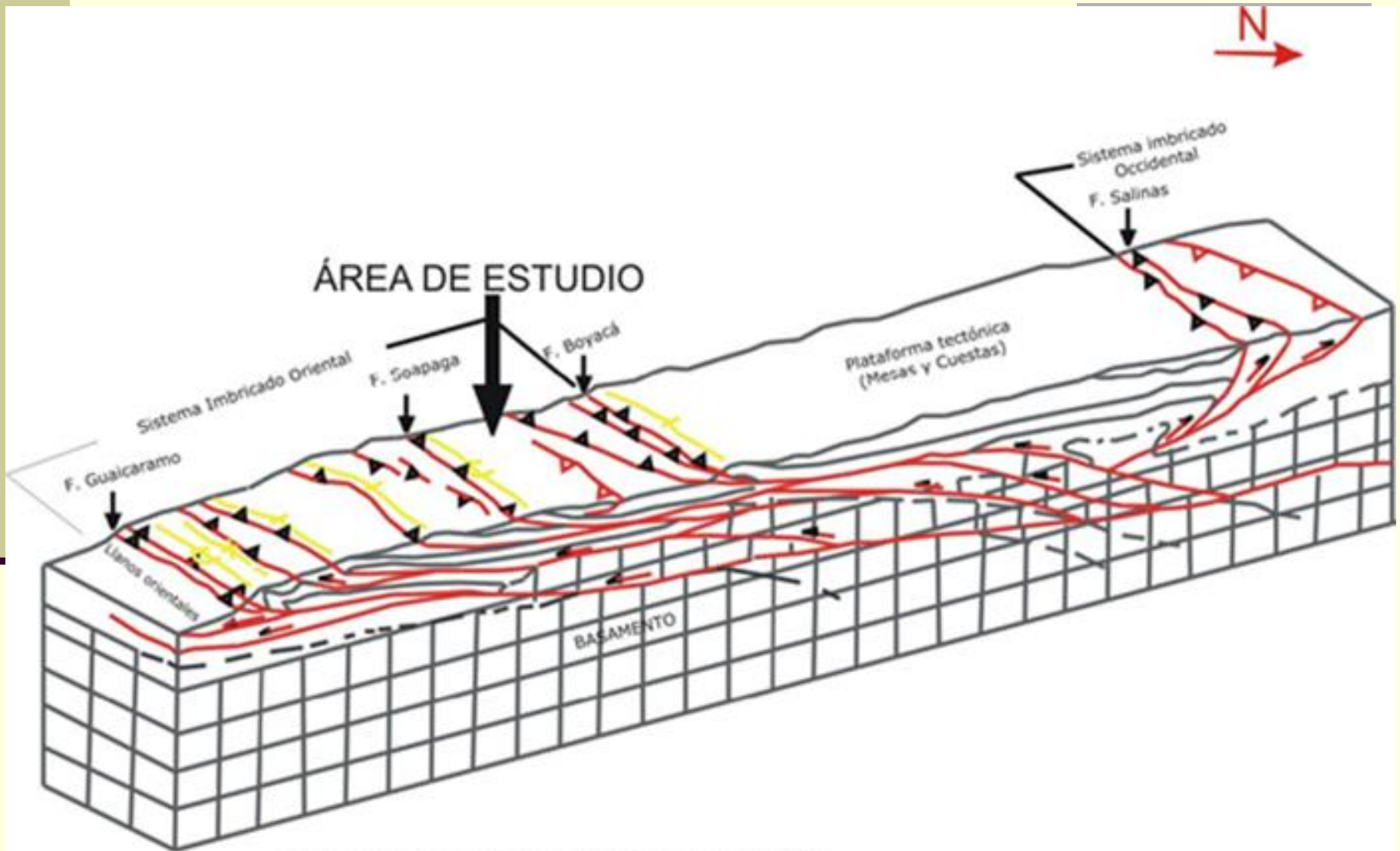
Modelo estructural de cordillera. Según Reyes (2001)
