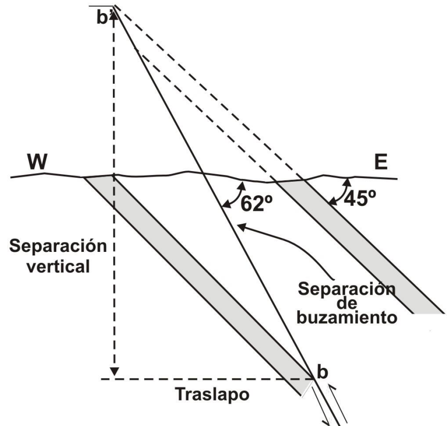
Perfil A - A'
