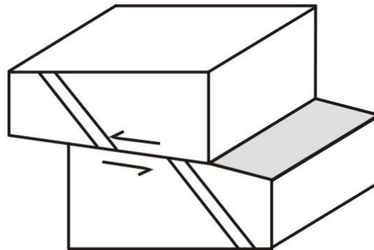
(e) cabalgamiento
