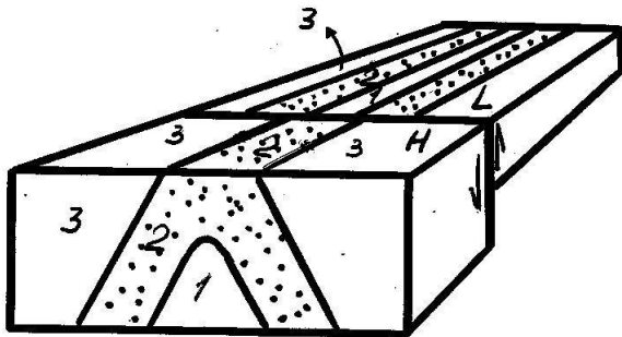
c) post erosión
